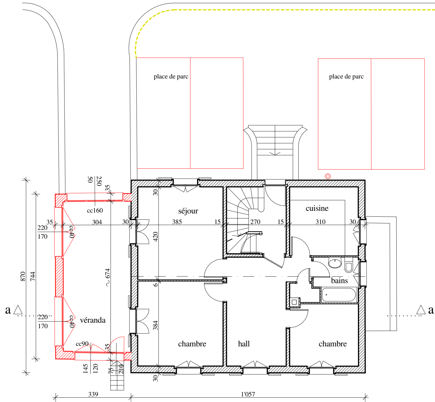
rez-de-chaussée
