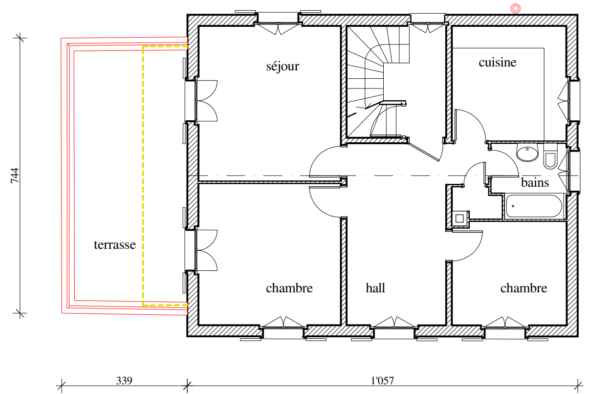
1er étage
